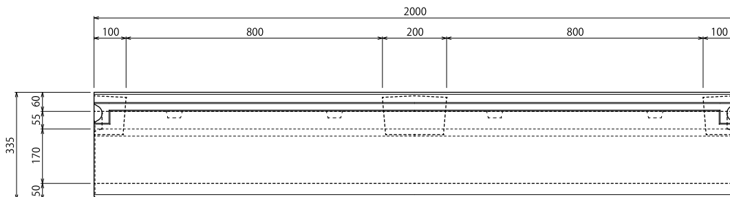
側面図
