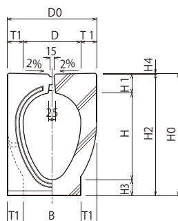
正面図
