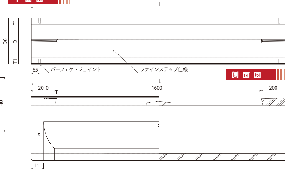
平面図
