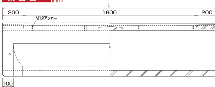
側面図
