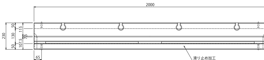
平面図
