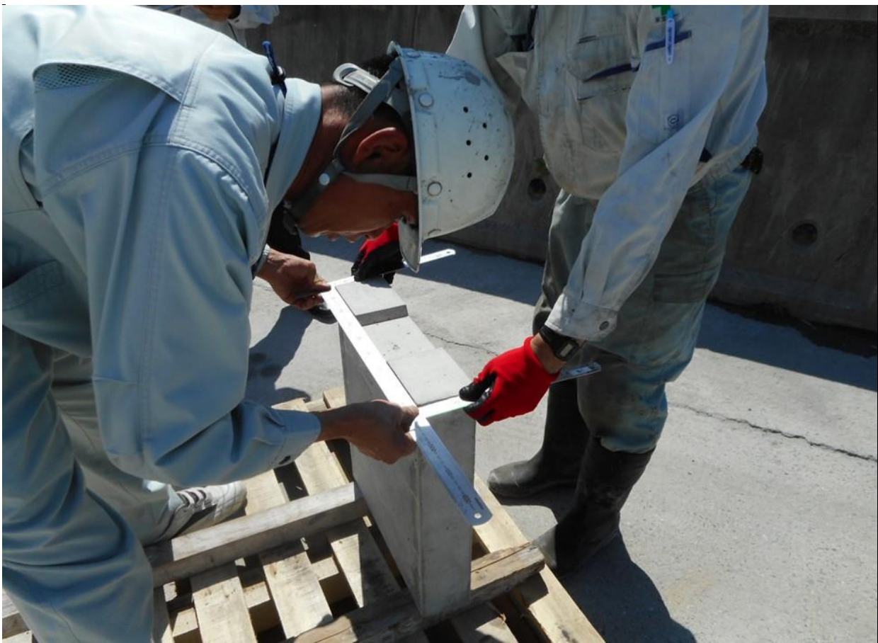
添付写真:落ちふた式U形側溝 ふた
