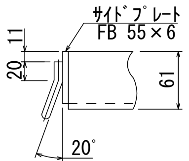
サイドプレートアンカー取付詳細
