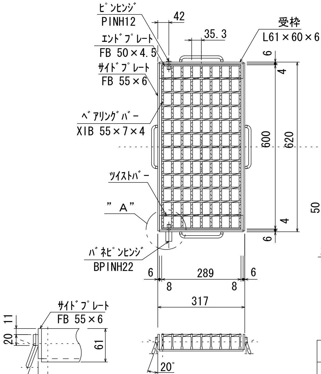
サイドプレートアンカー取付詳細
